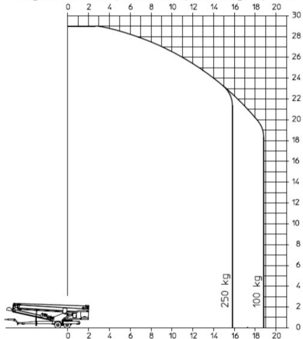
Arbeitsdiagramm Bühne / Werkdiagramm werkplatform / Diagramme de travail plate-forme / Operation diagram platform
